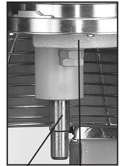
Arbre Boîtier du planétaire
