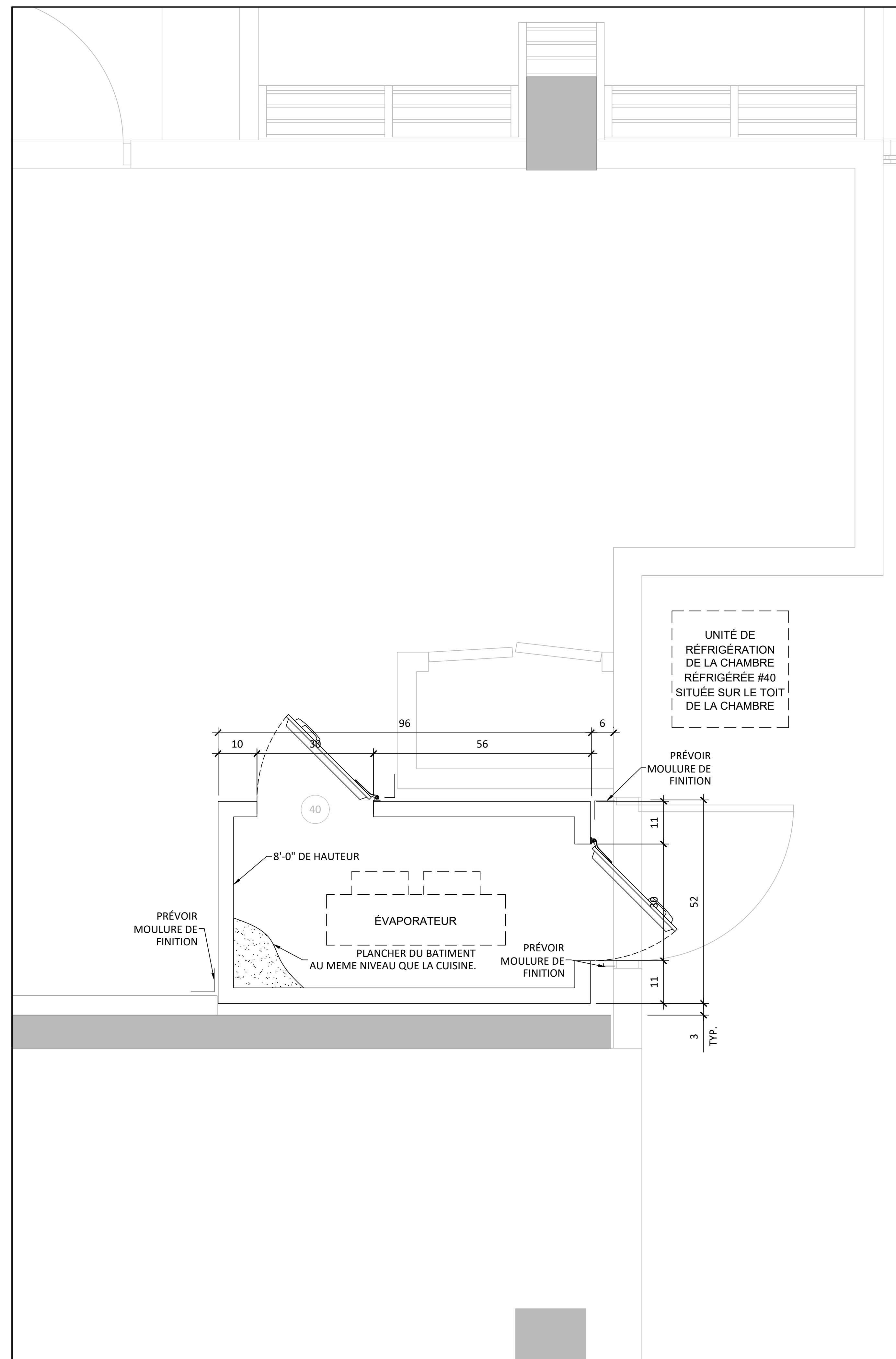
CHAMBRE RÉFRIGÉRÉE POUR DÉCHETS #40 ÉCHELLE: 1" = 1'-0"
