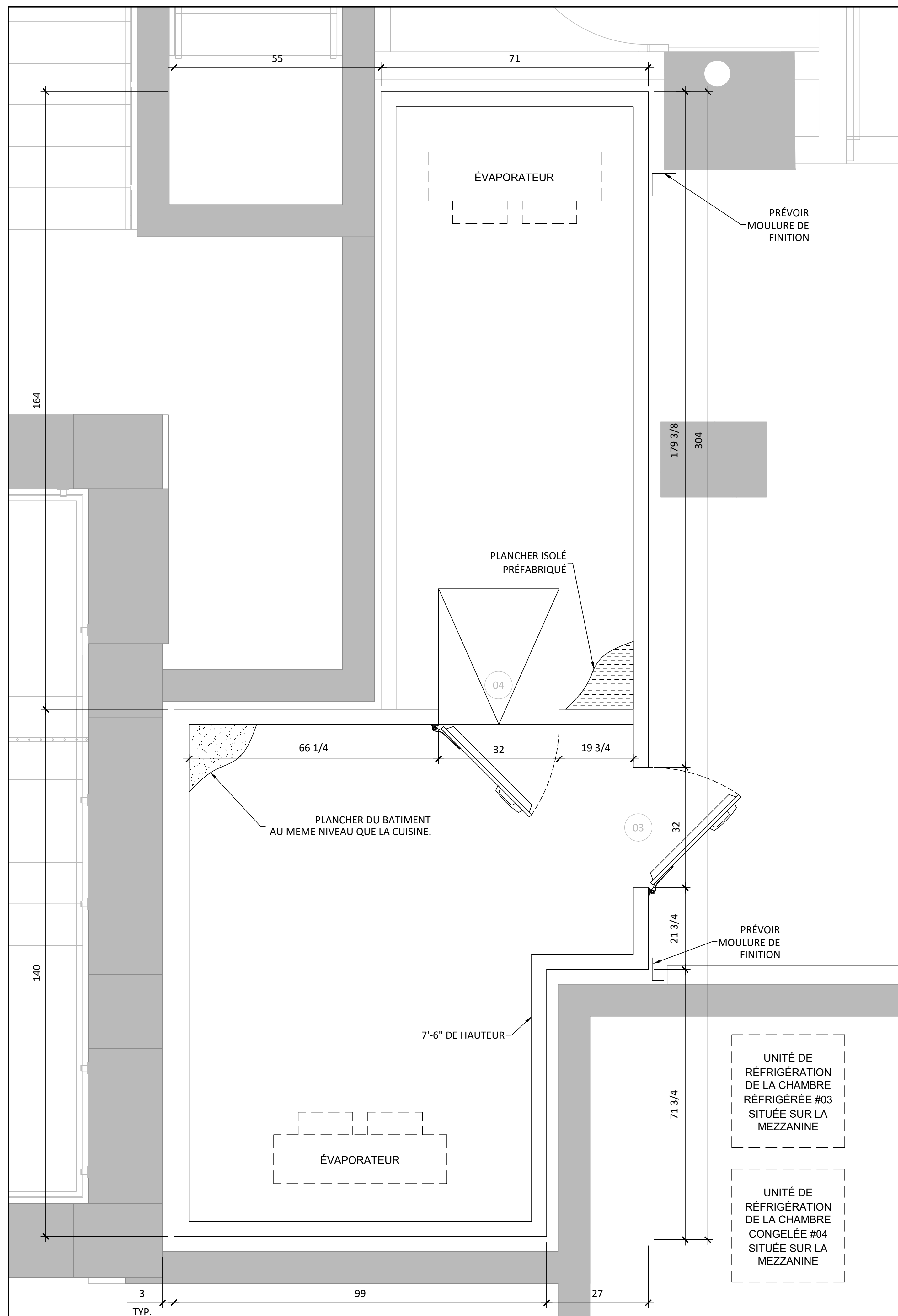
CHAMBRE RÉFRIGÉRÉ #03 & CHAMBRE CONGELÉ #04 ÉCHELLE: 3/4" = 1'-0"
